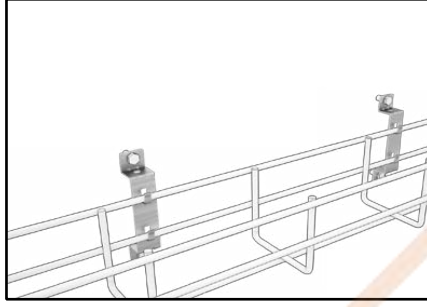
Taşıyıcı - Yandan Askı Elemanı / Hanger Side Support
