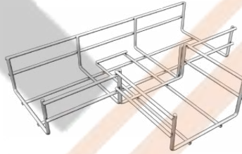
EK TKT ( W Genişlik )( H Yükseklik )( Tel Çapı )
