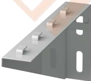
Tırnaklı Duvar Konsolu / Wall Bracket for Wire Mesh Cable Tray
